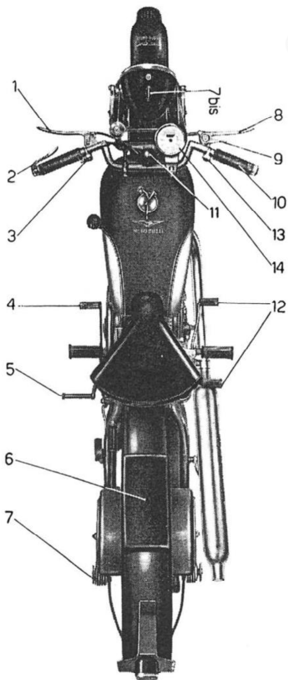
Fig. 3 - Comandi ed accessori
