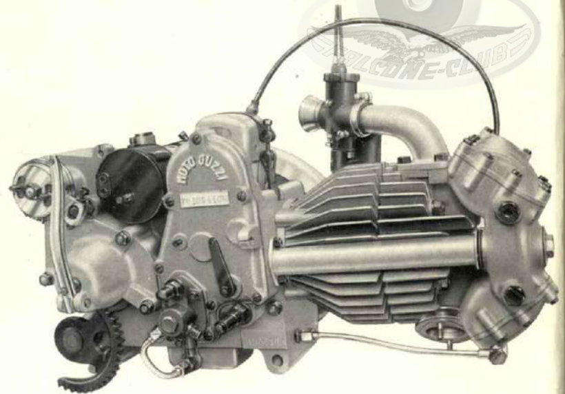
Fig. 4 - Lato destro (tipo Turismo)
