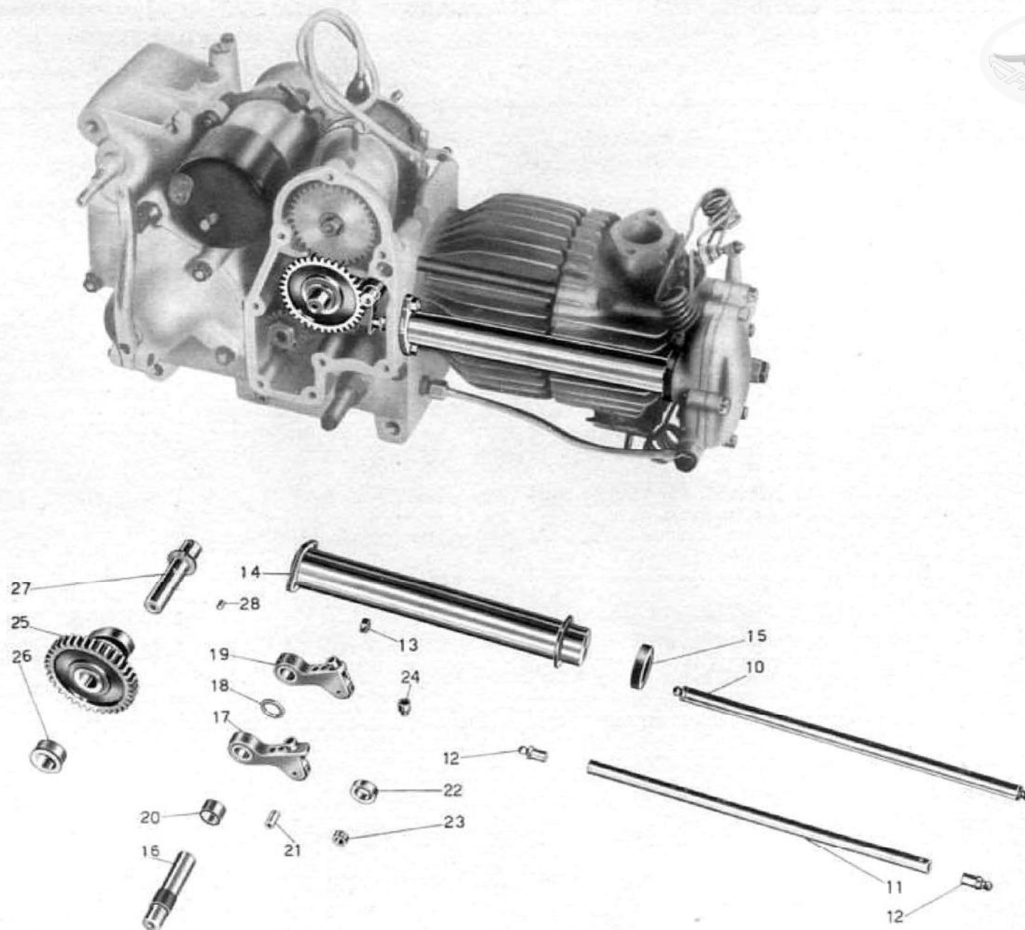
Tavola 4
