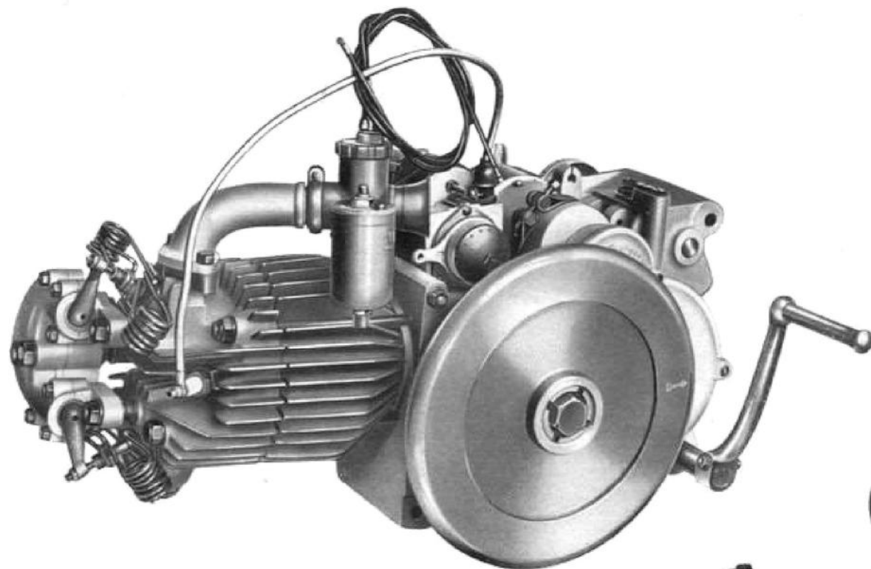
Fig. 4 - Lato volano
