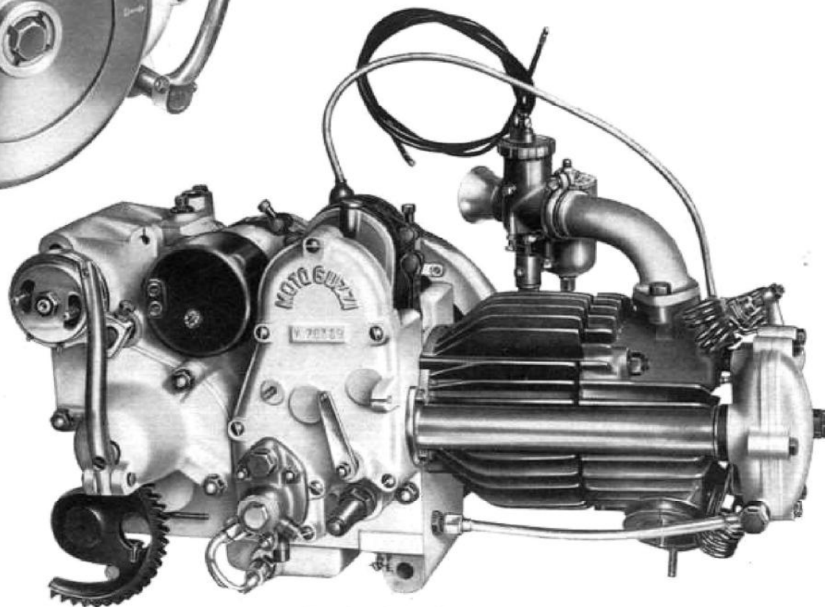
Fig. 5 - Lato distribuzione
